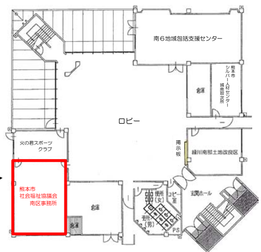
熊本市城南福祉センター平面図（1階）
